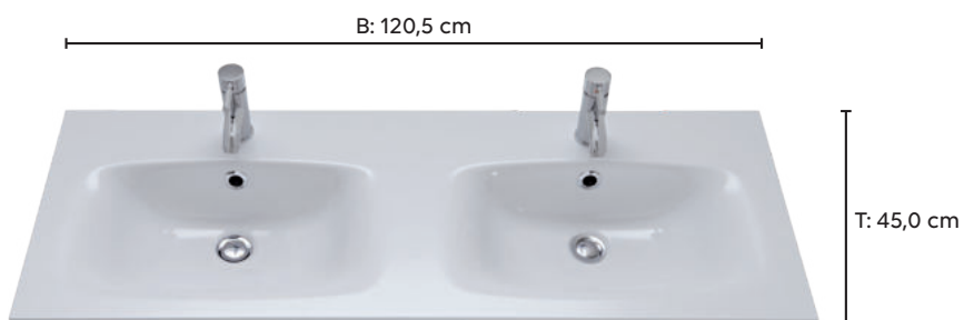
MWAZU12D Sichtbare Höhe: 1,5 cm, Beckenmaß: 2x B 56,0 cm x H 12,0 cm x T 30,0 cm
